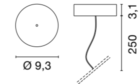
Rosone completo di cavo di alimentazione Ceiling rose with cable
