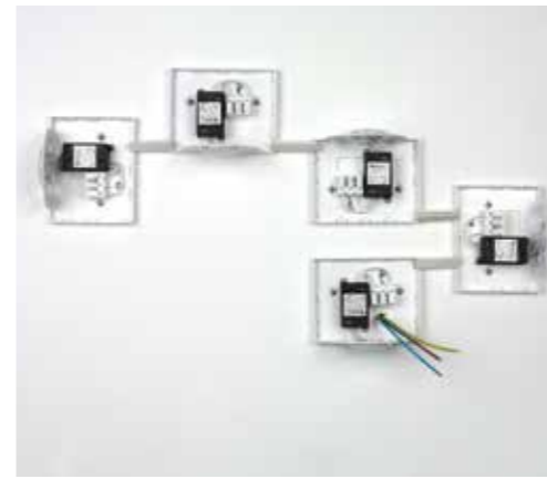
Fissaggio montature con uscita alimentazione da un solo punto luce e predisposizione collegamenti Installation of mounting plates starting from a single cable outlet
