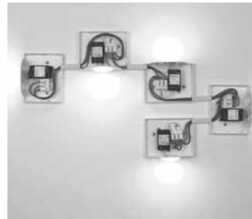
Realizzazione cablaggio passante tra le singole montature Realization of electrical connection between single units
